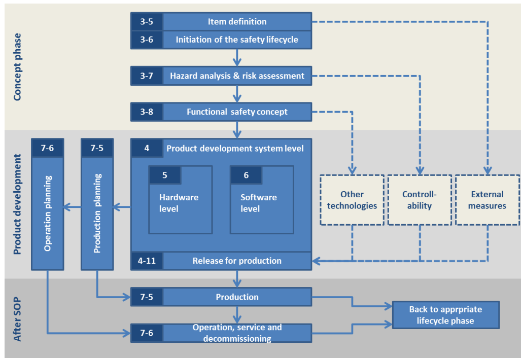
Abbildung 2: Sicherheitslebenszyklus 9
