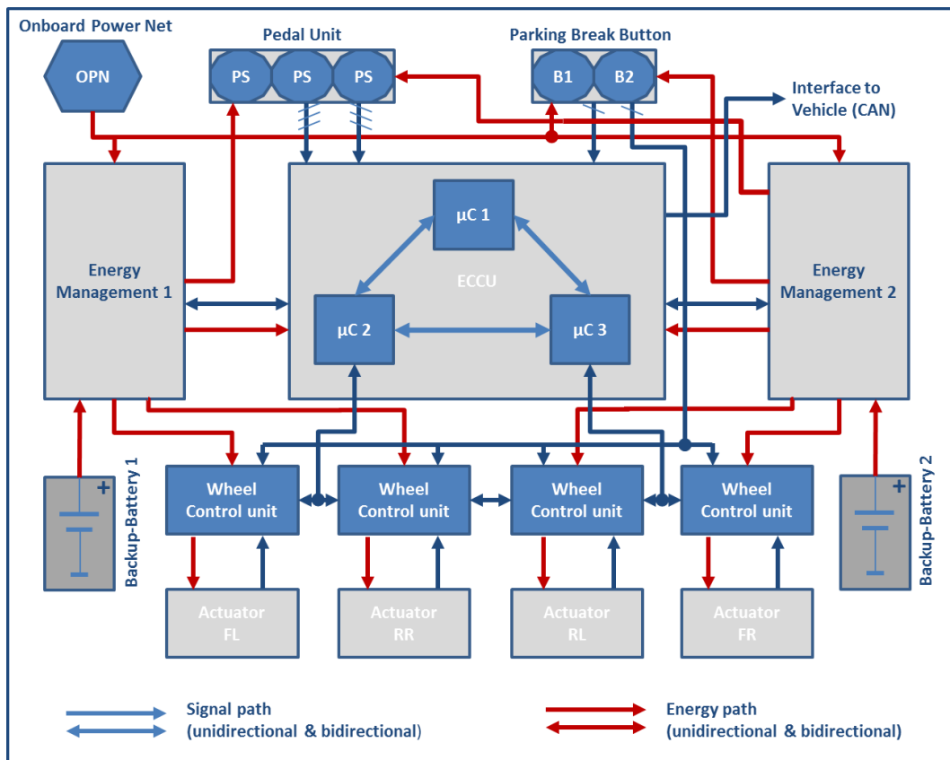
Abbildung 6: Systemarchitektur 26
