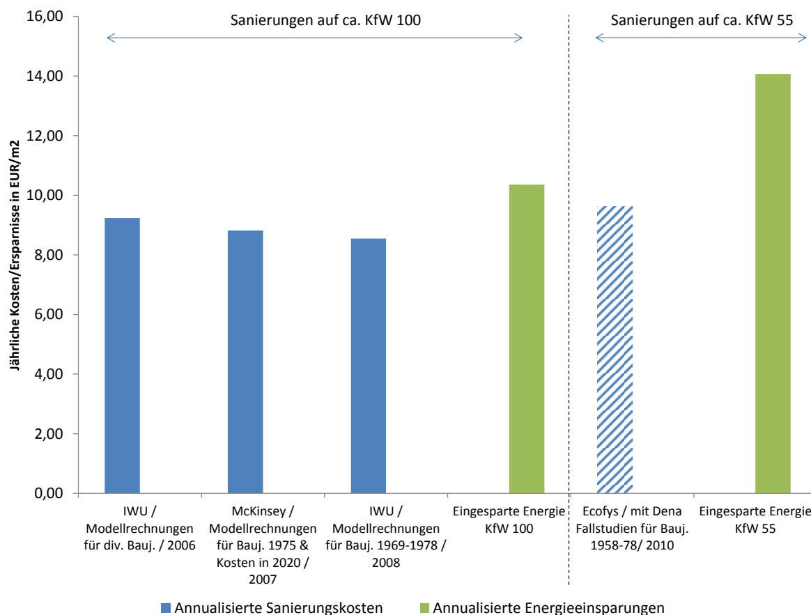
Abbildung 7: Kosten und Nutzen von Sanierungsmaßnahmen für EFHs (Schraffierte Flächen = ex-post Analysen). Annahme: Kredit über 20 Jahre mit 4% Zins, 1,5% Inflation, 7 Cent/kWh Endkundengaspreis (für Energiepreis siehe Anhang 5)
