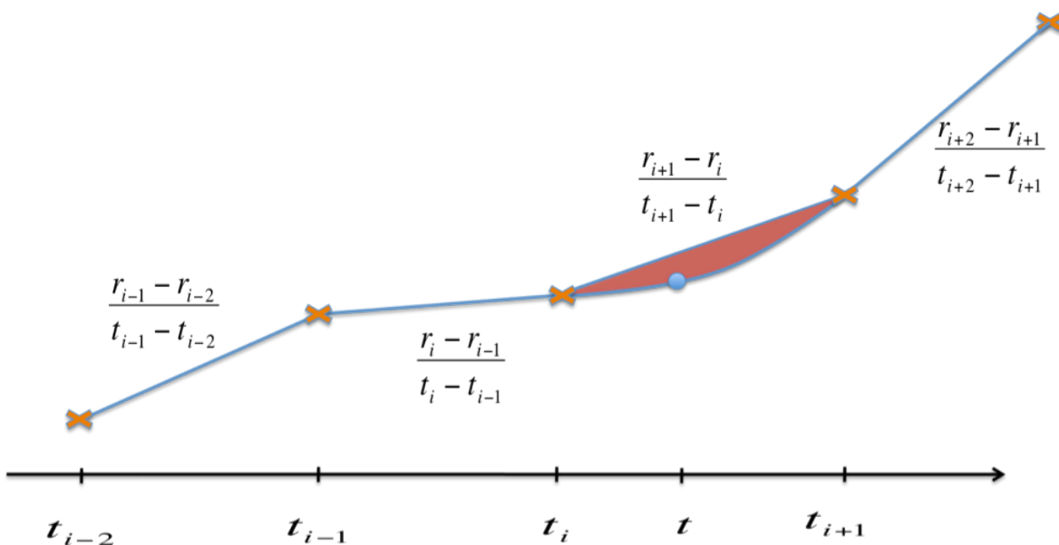
Abbildung 24, Funktionsweise der Approximation der cubic splines Interpolationsmethode
