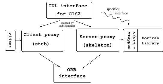
Fig. 3. Proxy pattern.
