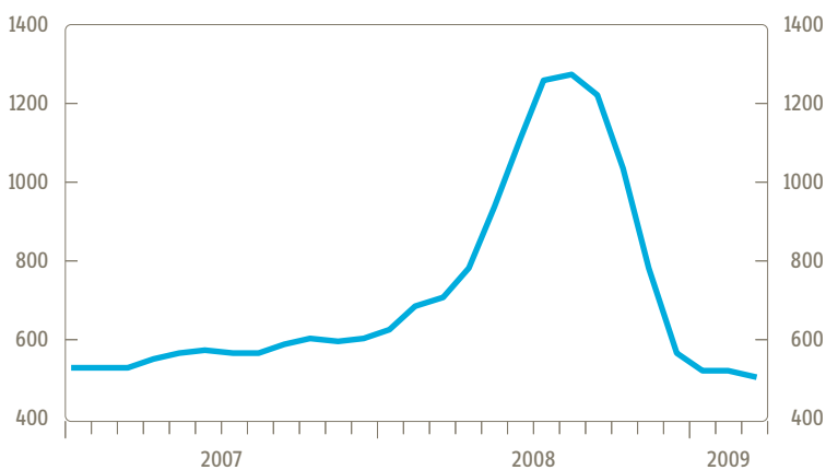
Schaubild 3 Stahlpreise 2007 bis 2009; Warmbreitband in $/t
