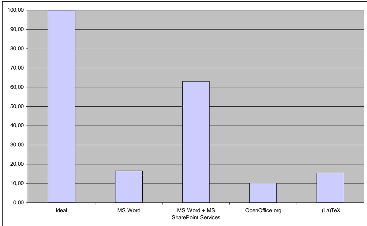
Abbildung 8: Verteiltes Arbeiten
