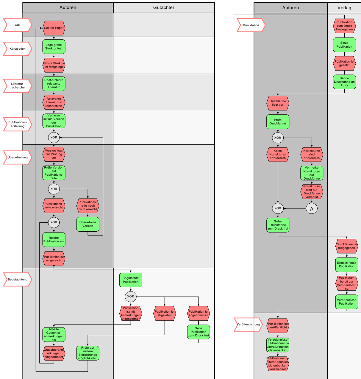
Abbildung 1: Publikationsprozess
