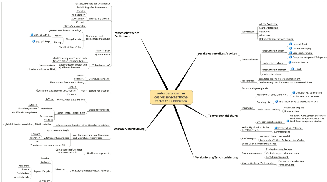
Abbildung 3: Mind Map
