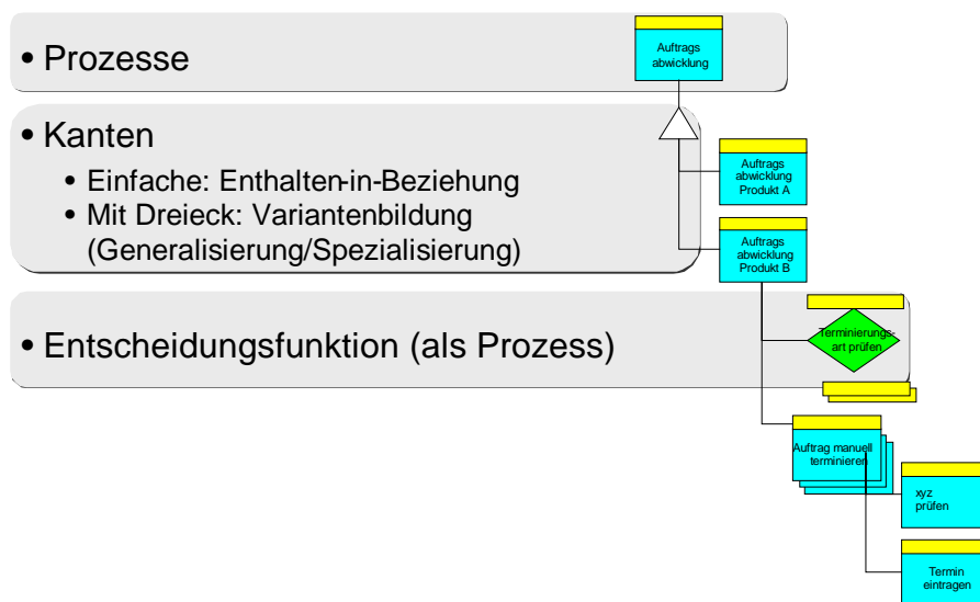
Abb. 3.7: Prozessbaum
