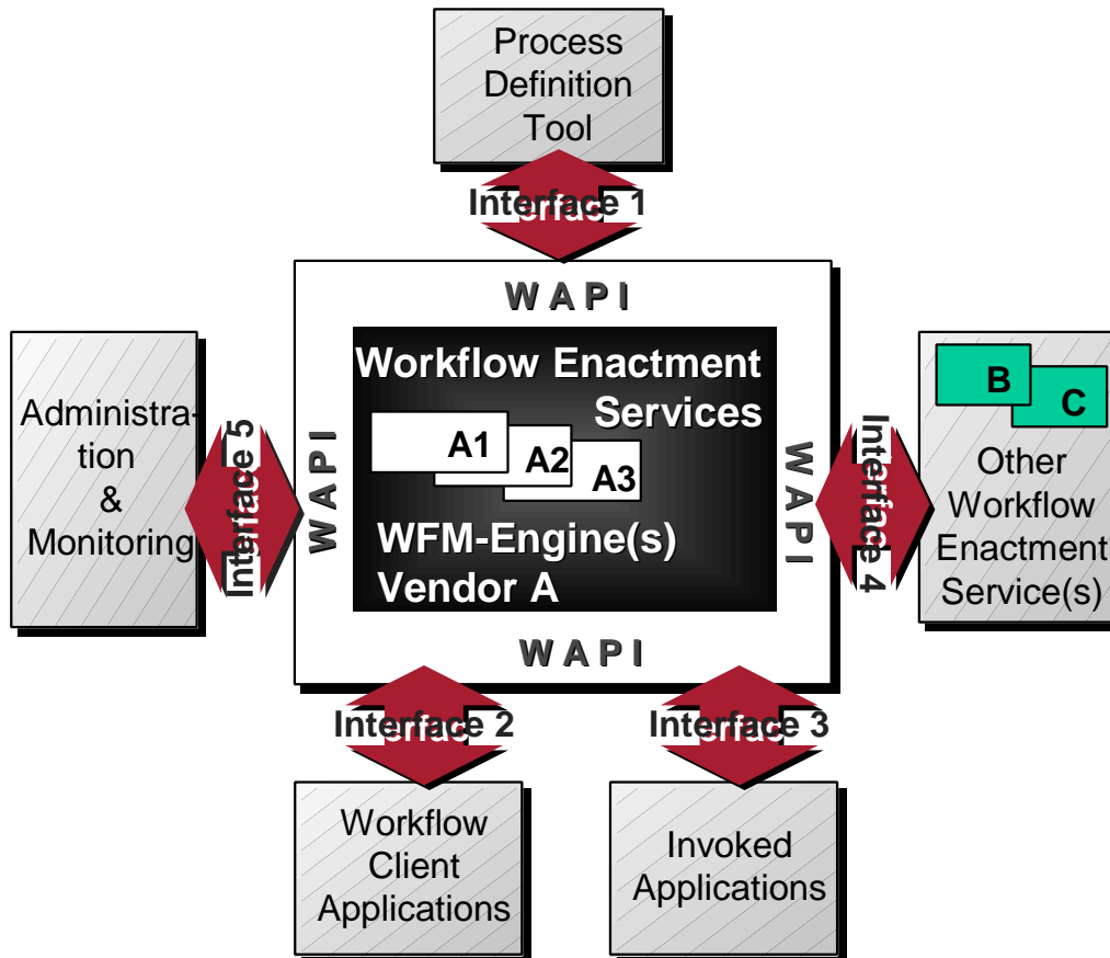
Abb. 5-2: Das Referenzmodell
