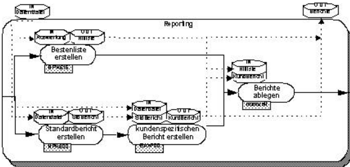
Abb. 3.3: Funktions-, Verhaltens-, Operations- und Informationsaspekt des Workflows 'Reporting'
