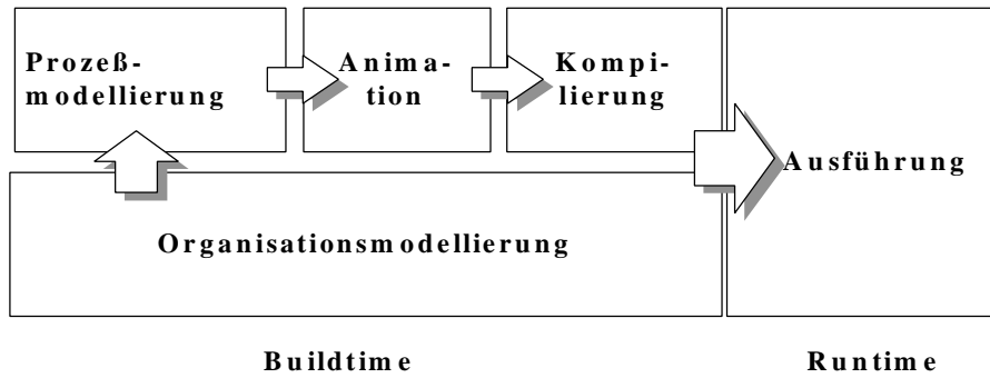
Abb. 6-2: FlowMark-spezifisches Vorgehensmodell
