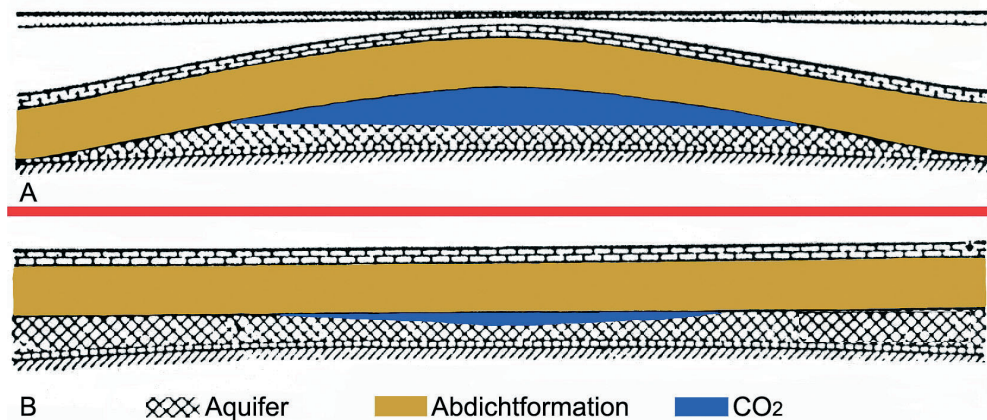
Abbildung 12: Geologische Voraussetzungen für eine stabile Speicherung Fall A: Stratigraphische und Strukturelle Falle, Fall B: Stratigraphische Falle (WI/GD 2006)
