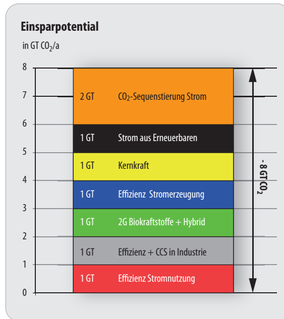
Abbildung 5: Mögliche zusätzliche CO 2 -Minderungsbeiträge gegenüber dem „Alternative Policy Scenario“ (APS) im Rahmen des „Beyond Alternative Policy Scenario“ (BAPS) für das Jahr 2030 (nach IEA 2006)
