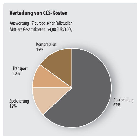
Abbildung 13: Verteilung der durchschnittlichen CCS-Kosten für Abscheidung, Kompression, Transport und Speicherung aus dem GESTCO-Projekt (nach GESTCO 2004)
