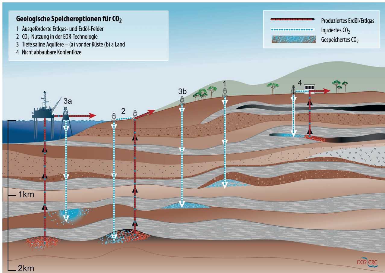
Abbildung 9: Mögliche geologische CO 2 -Speicheroptionen (nach IPCC 2005; Bild: CO2CRC)
