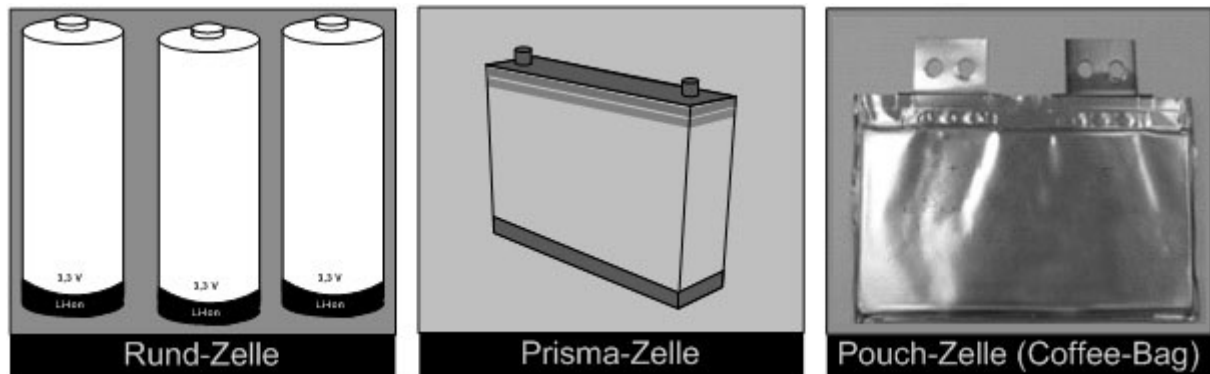
Abb. 4: Zelldesigns für die Verwendung in Elektrofahrzeugen [eigene Darstellung in Anlehnung an Saft12, Sb112, Wall11]
