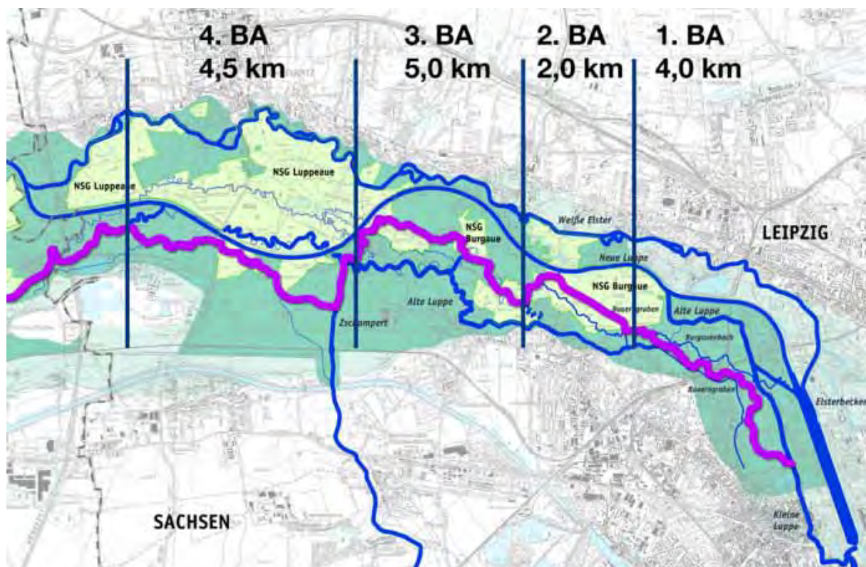
Abb. 7: Bauabschnitte
