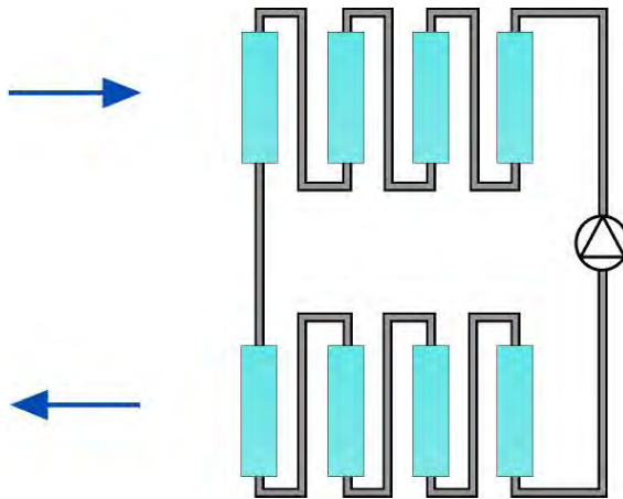
Abbildung 23: Kreislaufverbund Wärmetauscher 20
