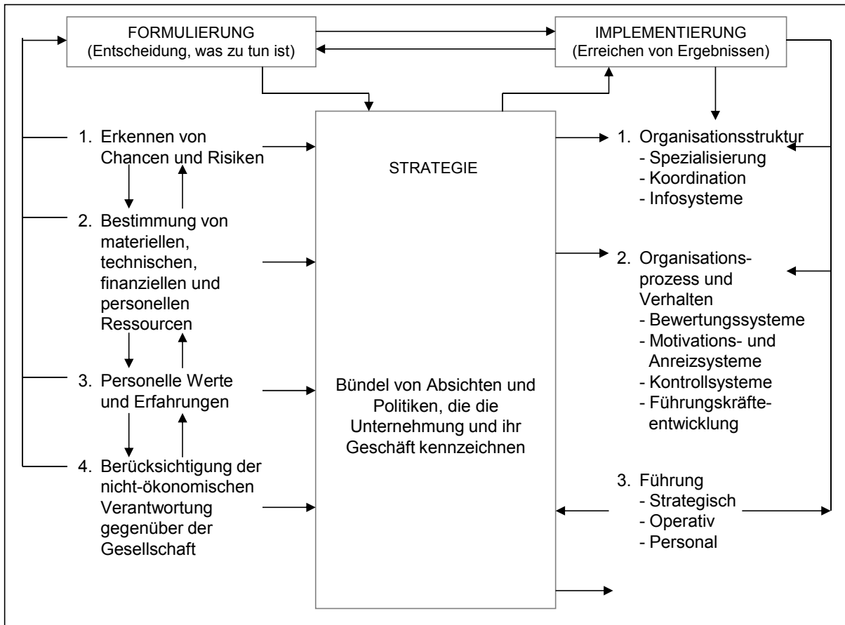
Abbildung 27: Modifiziertes LCAG-Schema 170
