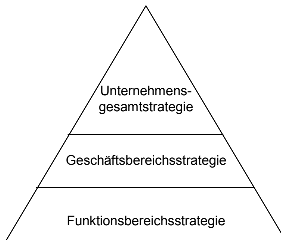
Abbildung 32: Strategiepyramide 183
