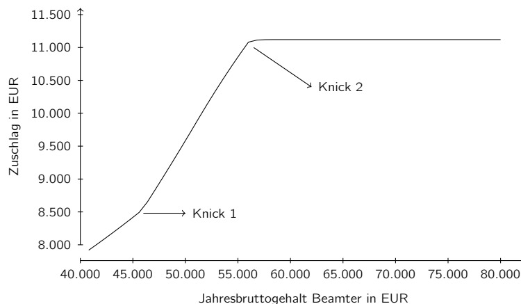
Abbildung 1: ohne Splittingvorteil
