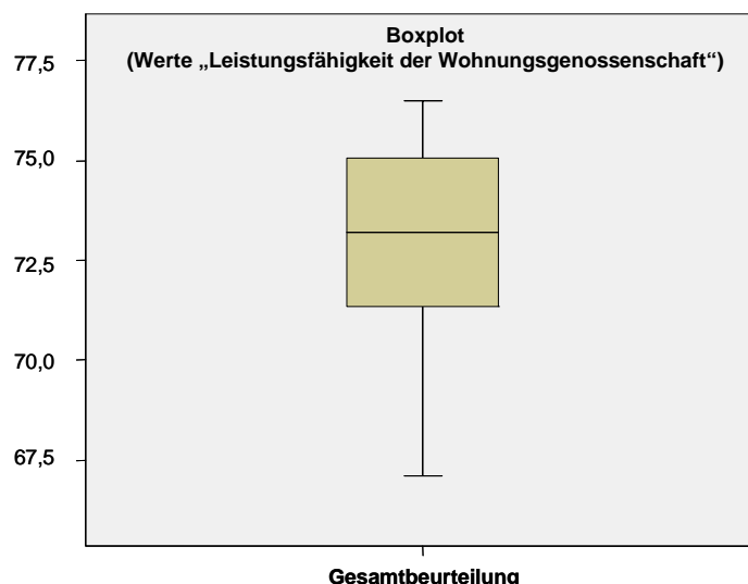
Abbildung 7: Boxplot „Leistungsfähigkeit“
