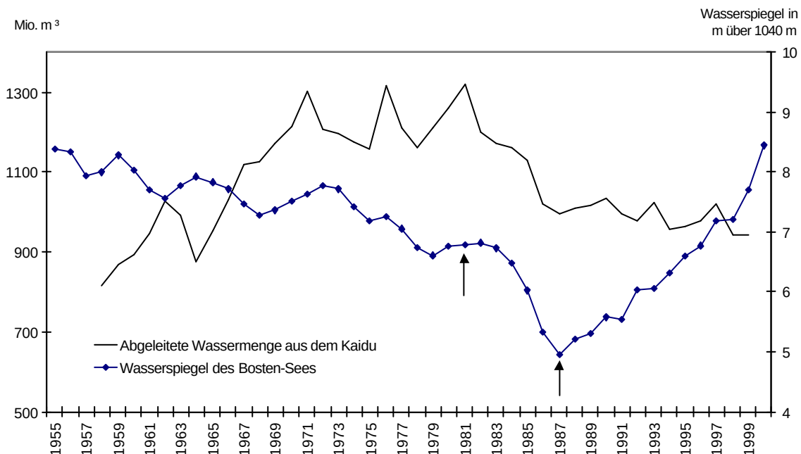
Abb. 5 Entwicklung des Wasserspiegels des Bosten-Sees und der abgeleiteten Wassermenge aus dem Kaidu 1956-2000
