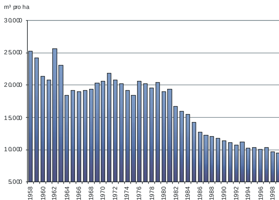
Abb. 13: Entwicklung des Wasserverbrauchs in m³ pro ha Bewässerungsfläche im Einzugsgebiet des Kaidu 1958 – 1999
