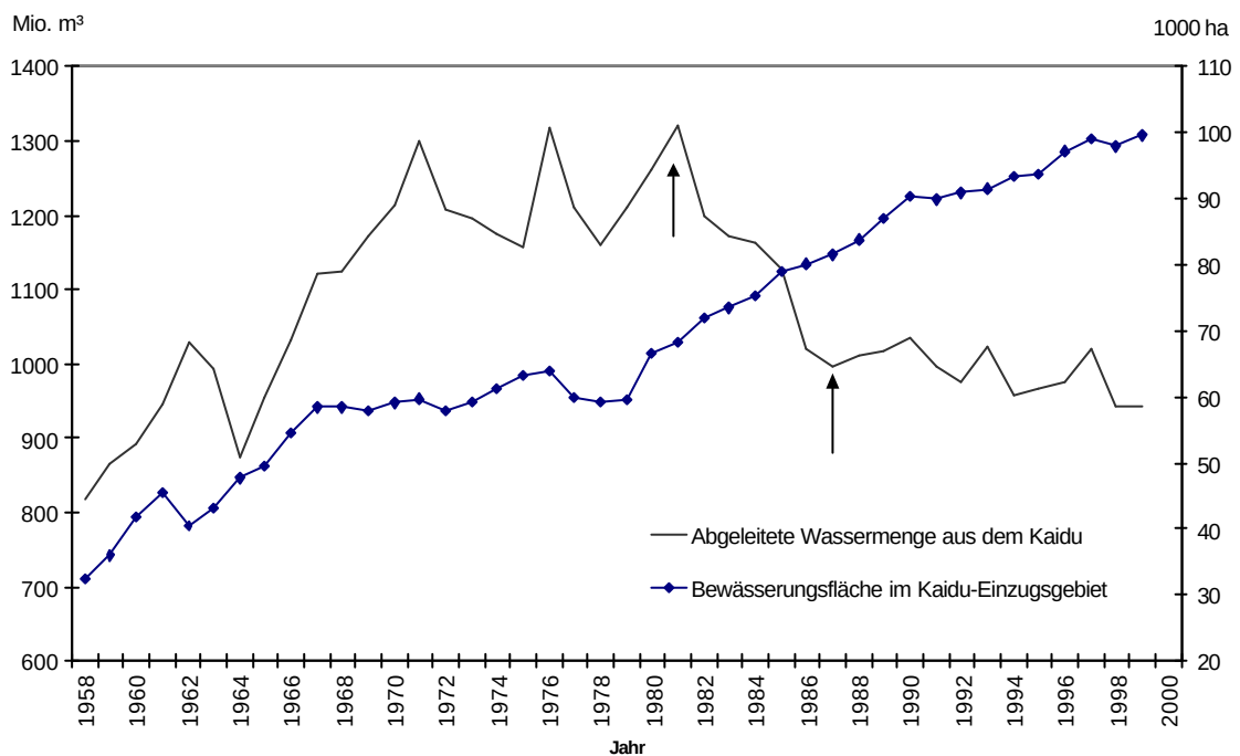
Abb. 6 Entwicklung der Bewässerungsfläche und der abgeleiteten Wassermenge für Bewässerungszwecke aus dem Kaidu 1958 - 1999
