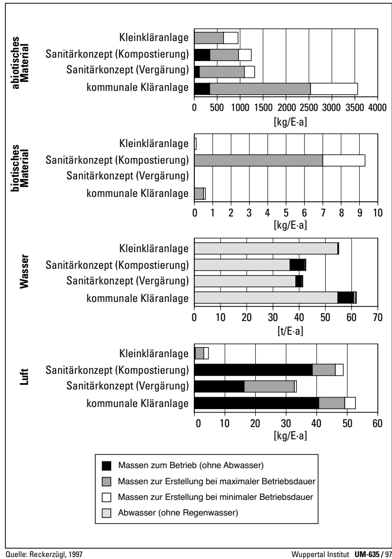
ABB. 5. Vergleichende Materialintensitäts-Analyse verschiedener Abwasserbehandlungssysteme (Reckerzügl und Bringezu 1998). Varianten Nr. 1 – 4 von unten nach oben angegeben (s. Text).
