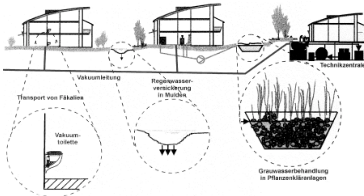
ABB. 4. Stoffstromseparation und Vakuumsystem zur semi-zentralen Sammlung und Behandlung von Siedlungsabwasser (Quelle: Otterpohl-Wasserkonzepte, siehe auch Otterpohl 1998).
