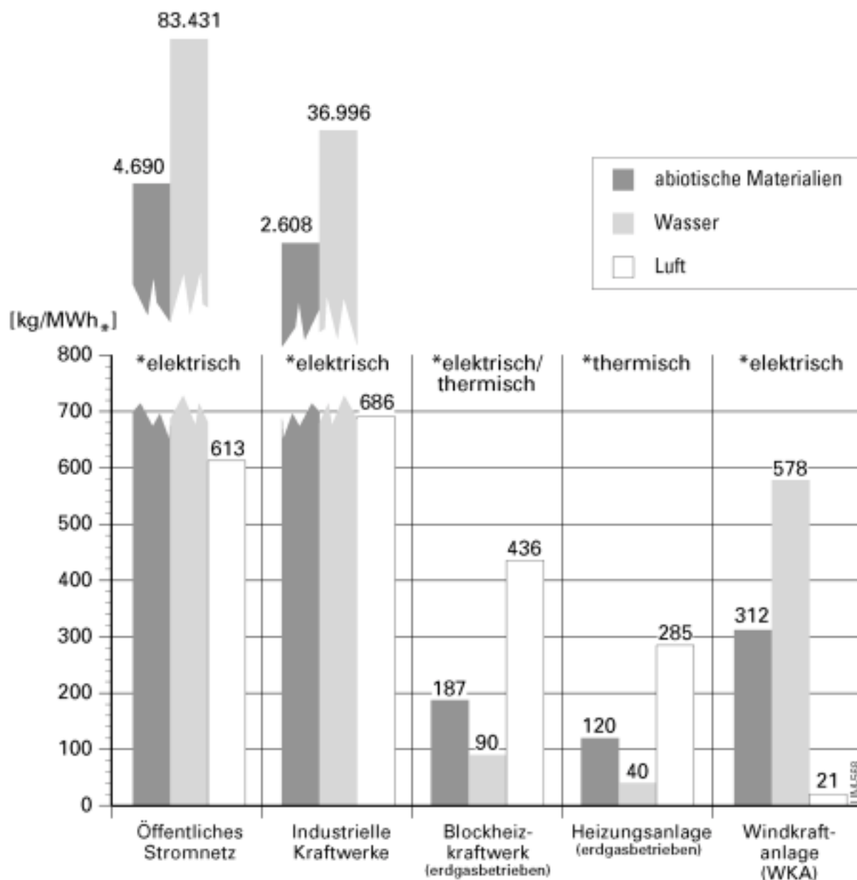
ABB.3. Die Materialintensität verschiedener Energieversorgungssysteme (Manstein in Liedtke et al. 1996 sowie zusätzliche Berechnungen).
