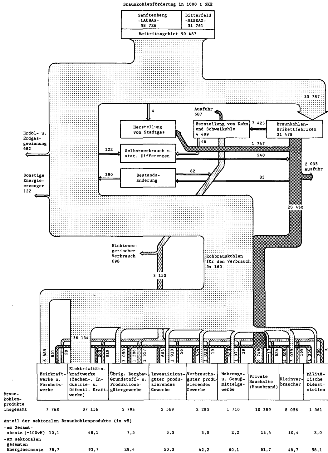
Schaubild 4 - Flußbild der Braunkohlenversorgung in der DDR 1989 (1000 t SKE)
