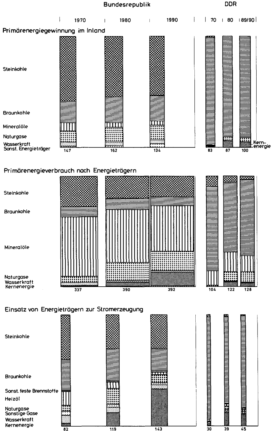
Schaubild 1 - Struktur des Energiesektors der DDR und der Bundesrepublik 1970, 1980 und 1989/90
