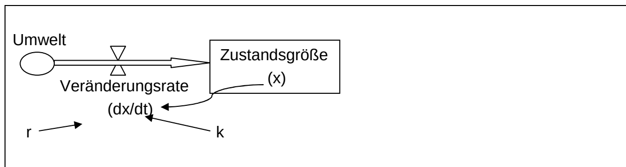
Abb. 1: Darstellung des dynamischen Systems für ein logistisches Wachstum
