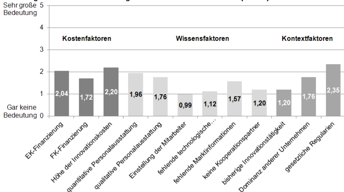
Abbildung 5: Mittlere Bedeutung der Innovationshemmnisse (n=224)
