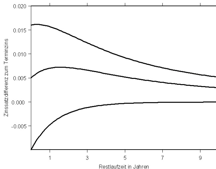
Abbildung 1: Formen der Zinsstruktur im stationären Ein-Faktor-Modell
