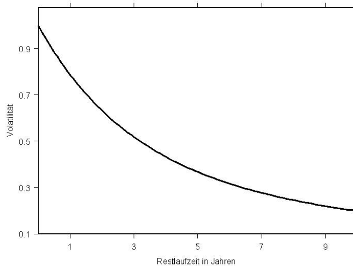
Abbildung 2: Fristigkeitsstruktur der Volatilität im stationären Ein-Faktor-Modell
