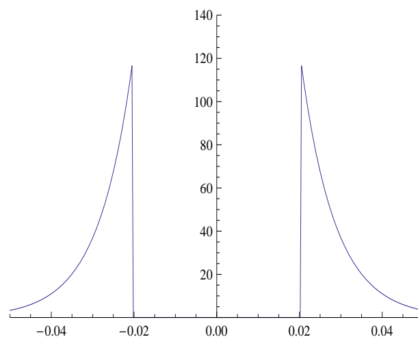
Abbildung 2: Displaced Double-Exponential Dichte von E mit Parametern \kappa = 2,019\% , \eta = 0,827\%
