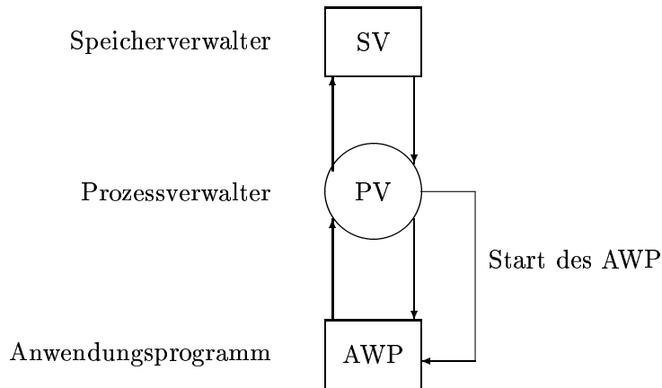
Abbildung 6: "Drehscheibe" Prozessverwalter
