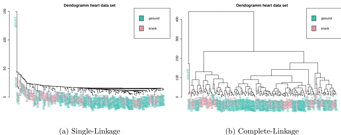
Abbildung 13: Dendrogramme der hierarchischen Verfahren
