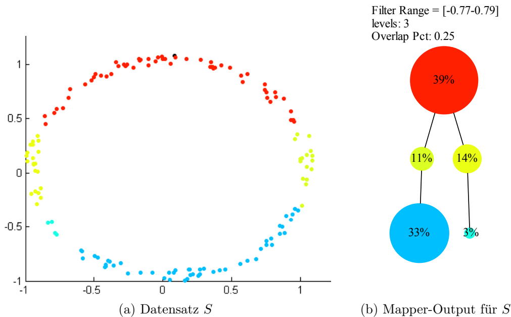
Abbildung 16: Reproduktion der Abbildung 16 (vgl. Nastansky (2019), S. 27) mit der Mapper-Software. Als Filter dient die Funktion f(x, y) = y . Der Homotopietyp von \mathbb{X} wird hier nicht erkannt.
