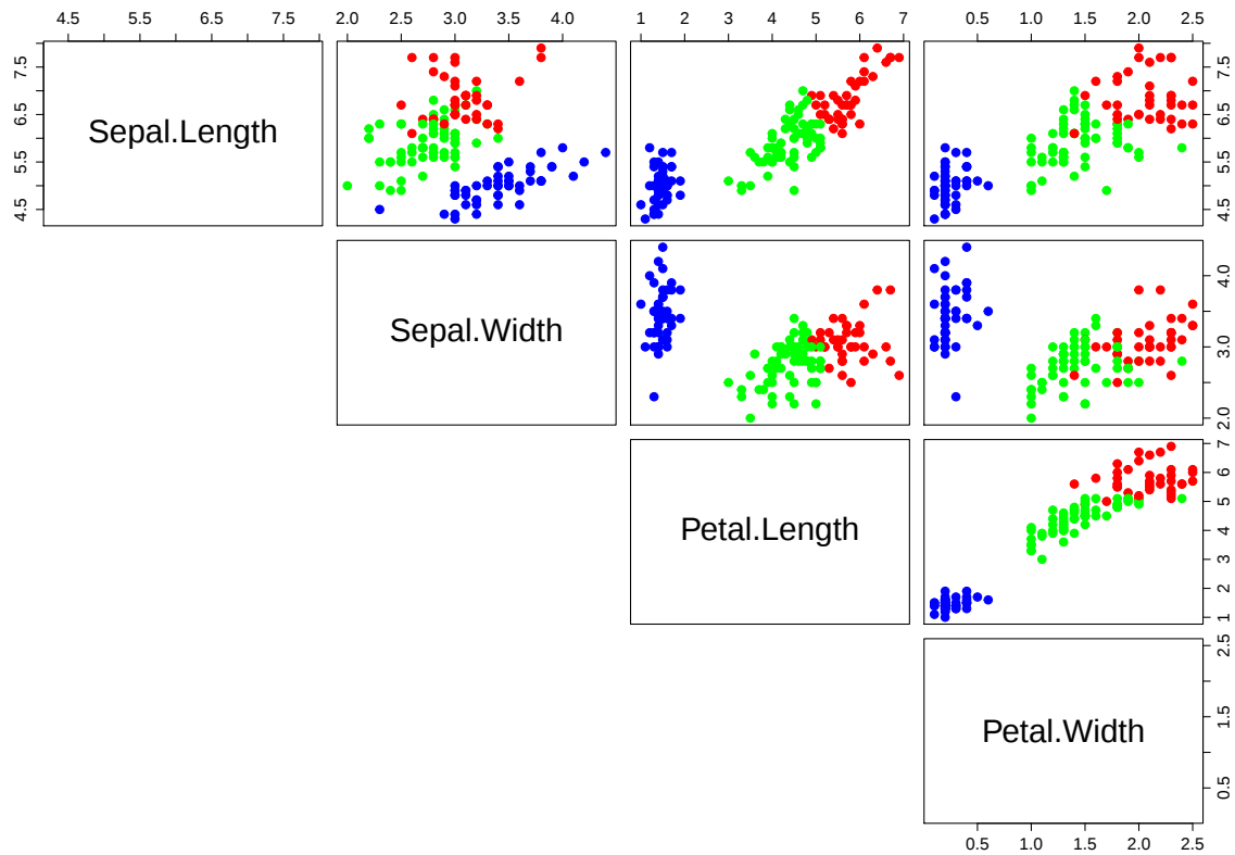
Abbildung 5: K -Means für den Iris Flower-Datensatz mit K = 3
