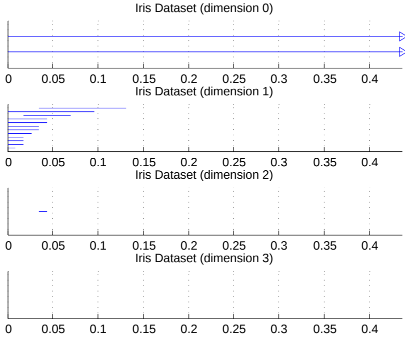
Abbildung 9: Persistente Homologie für den Iris Flower-Datensatz
