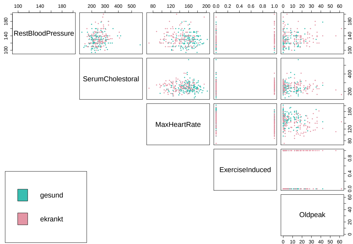
Abbildung 12: Heart Disease-Datensatz
