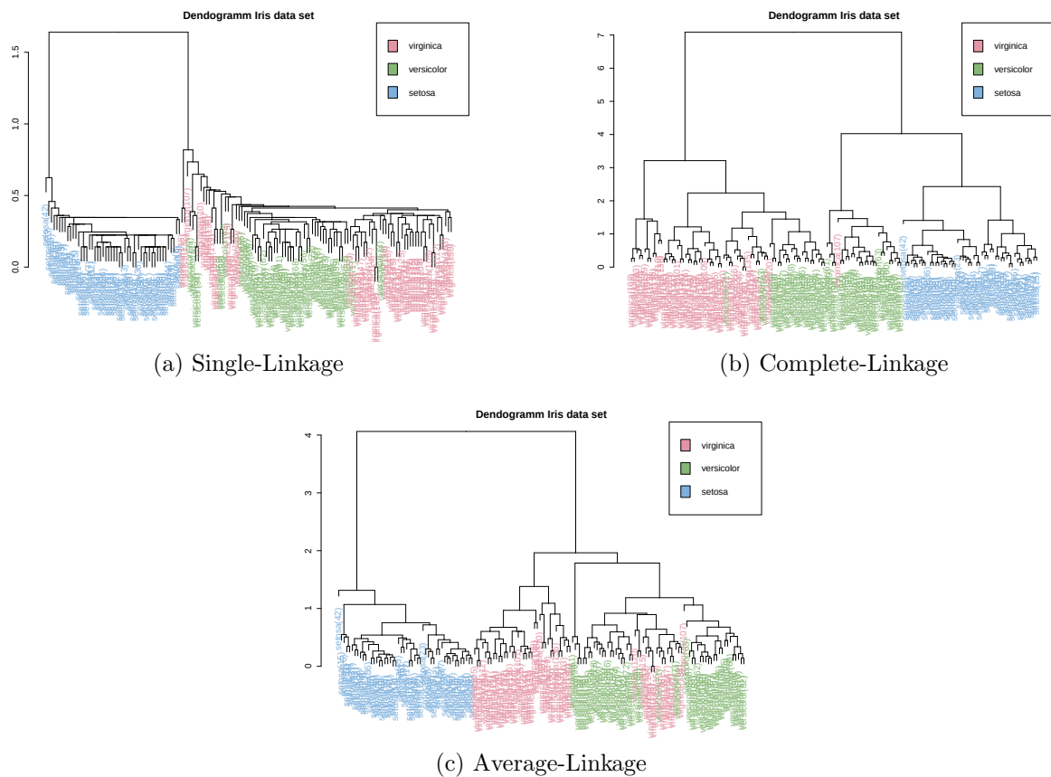
Abbildung 6: Dendrogramme der hierarchischen Verfahren
