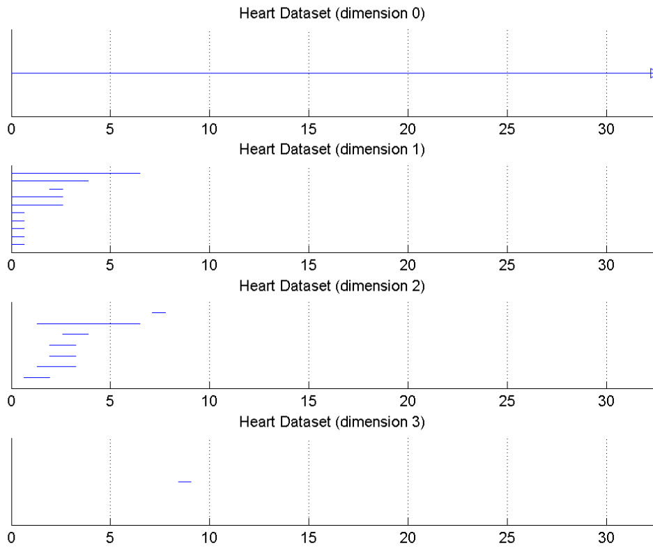
Abbildung 14: Persistente Homologie für den Heart Disease-Datensatz
