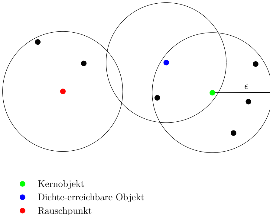
Abbildung 2: Arten von Punkten im DBSCAN Algorithmus ( MinPts = 6 )
