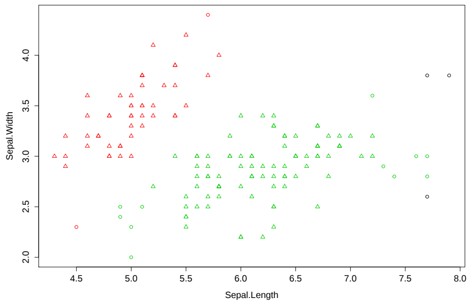
Abbildung 8: Beispiel Output des DBSCAN für den Iris Flower-Datensatz
