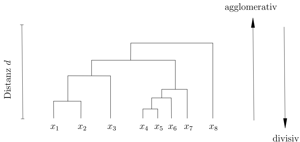
Abbildung 1: Dendrogramm der hierarchischen Clusteranalyse
