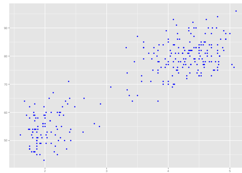
(a) Datensatz S
