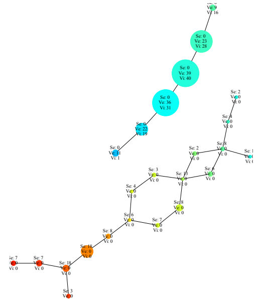
(d) Mapper(f^{-1}(\mathcal{V}(15, 0.95), \mathcal{C}))
