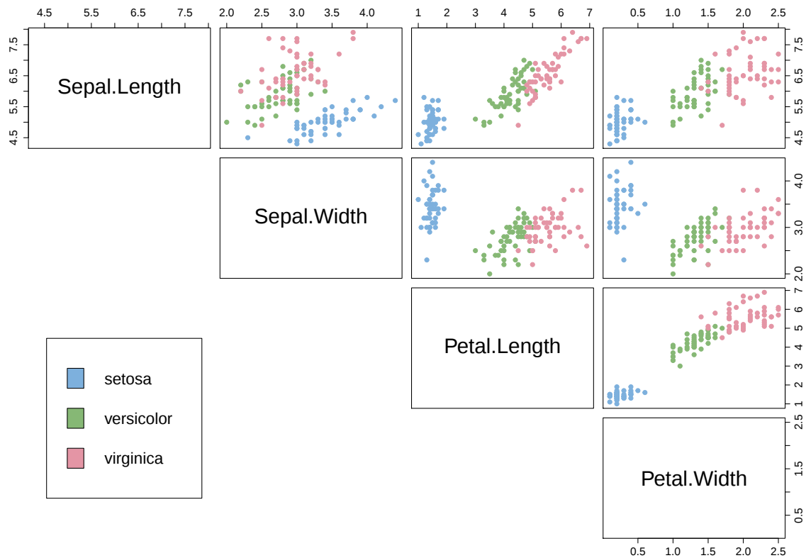
Abbildung 4: Iris Flower-Datensatz
