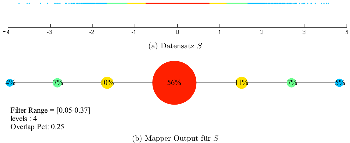
Abbildung 19: Reproduktion der Abbildung 17 mit der Mapper-Software. Als Filter dient hier die Standardnormalverteilung f(x) = \frac{1}{\sqrt{2\pi}} e^{-\frac{x^2}{2}} . In (a) ist wieder der Datensatz S und in (b) der Mapper-Output zu sehen.
