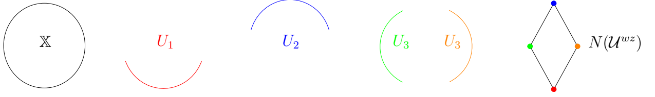
Abbildung 15: Überdeckung \mathcal{U}^{wz} von S^1 und dessen Nerv
