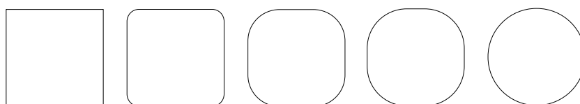
Abbildung 2: Homotopieäquivalenz zwischen einem Kreis und einem Quadrat
