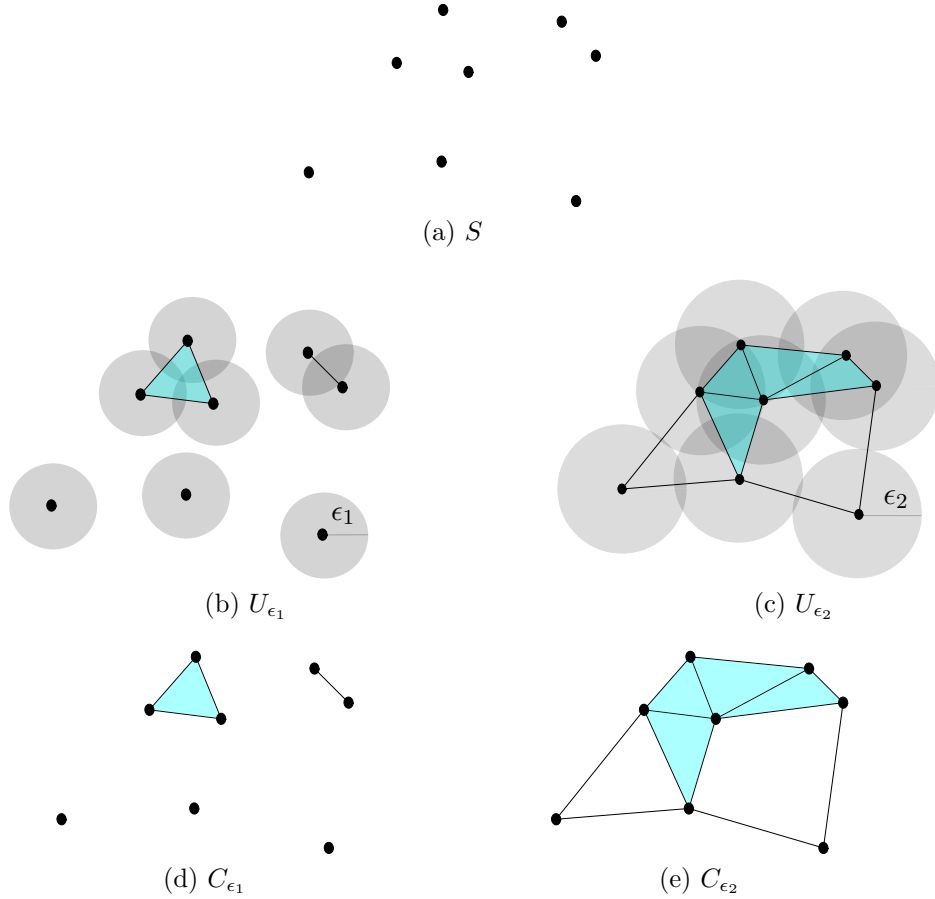
Abbildung 4: Punktwolke S , Überdeckungen U_{\epsilon_1} , U_{\epsilon_2} , sowie dazugehörige Čech-Komplexe C_{\epsilon_1} und C_{\epsilon_2}
