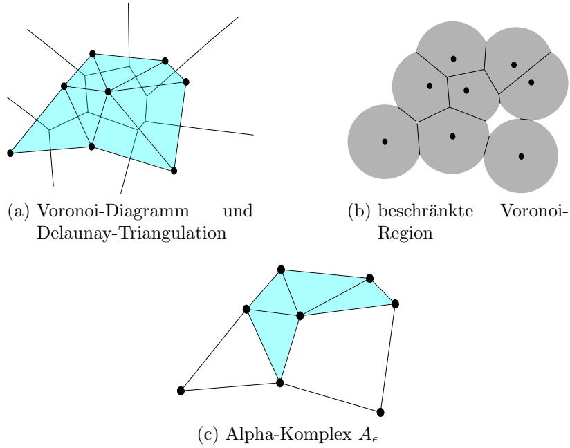
Abbildung 5: Voronoi-Diagramm, Delaunay-Triangulierung sowie beschränkte Voronoi-Region und Alpha-Komplex für die Punktwolke S
