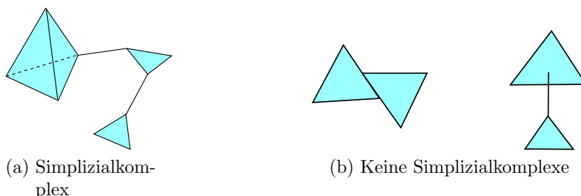
Abbildung 3: Beispiel und Gegenbeispiele für Simplicialkomplexe
