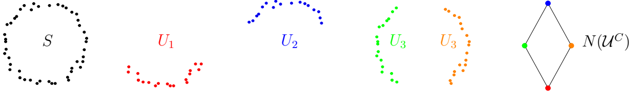
Abbildung 16: Überdeckung \mathcal{U}^C von S und deren Nerv
