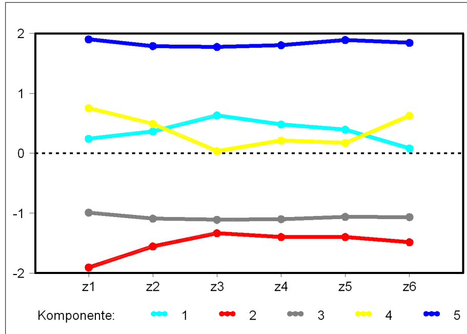
Abbildungung 8: Kompositionsabweichungsdiagramm (zu Tab. 1) (Verbindungen zwischen den Punkten für bessere Lesbarkeit)
