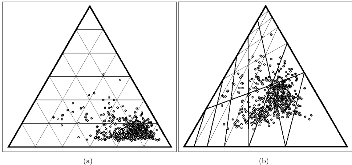
Abbildung 4: S^3 – Dreiecksdiagramm (Hilfslinien alle 16,6 %)
