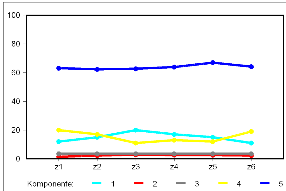
Abbildung 7: Kompositionen zu 100 % (zu Tab. 1)
