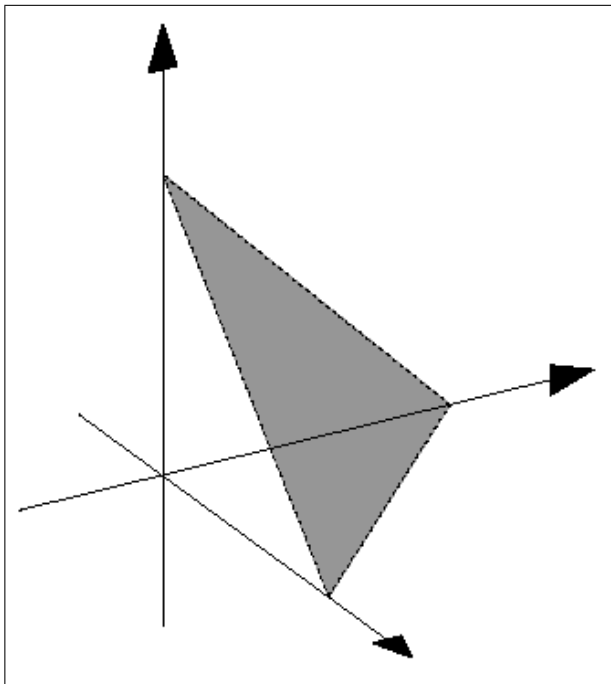
Abbildung 1: Simplex S^3 \subsetneq \mathbb{R}^3 – ein gleichseitiges Dreieck
