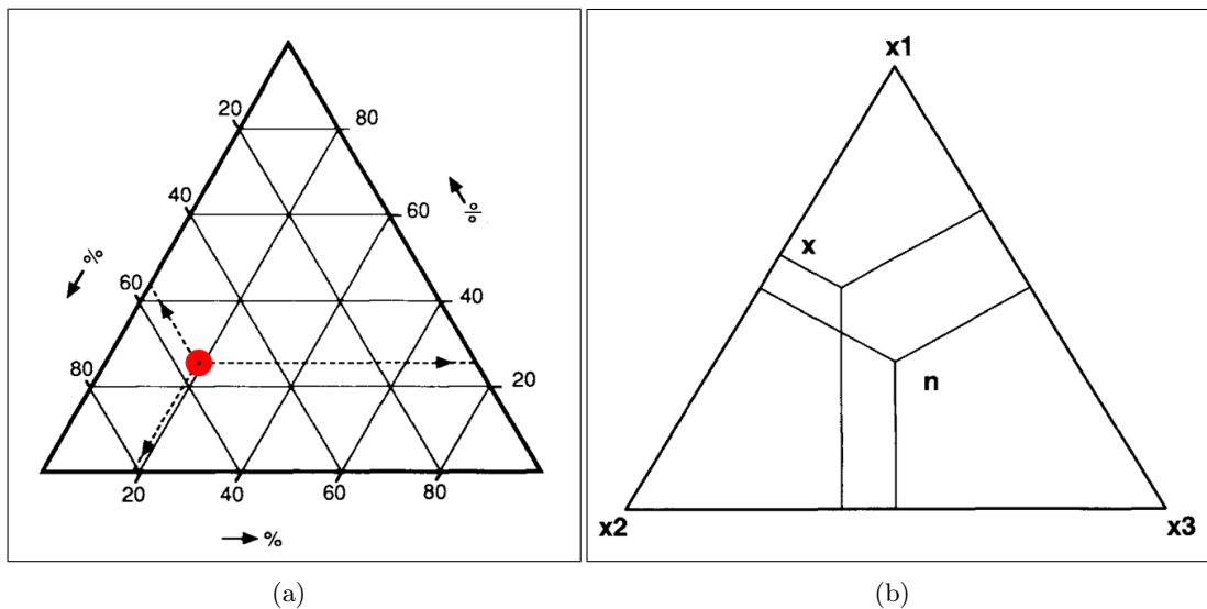
Abbildung 3: S^3 – Kompositionen im Dreiecksdiagramm
