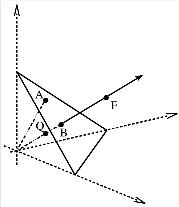
Abbildung 2: Simplex S^3 als Äquivalenzklasse:
