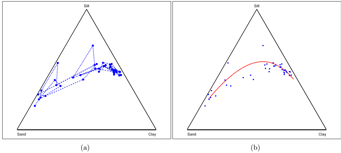
Abbildung 5: Sedimente als Kompositionen aus Sand, Schluff (silt) und Lehm (clay) in verschiedenen Tiefen eines arktischen Binnensees (a) Messdaten (verbunden in Reihenfolge der Tiefe unter Wasseroberfläche) (b) Regression mit \log(\text{Tiefe}) als Regressor (siehe Text)
