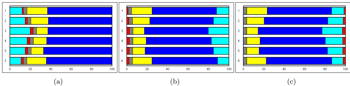
Abbildung 6: Kompositionen zu 100 % (Tab. 1) – Reihenfolge der Komponenten
