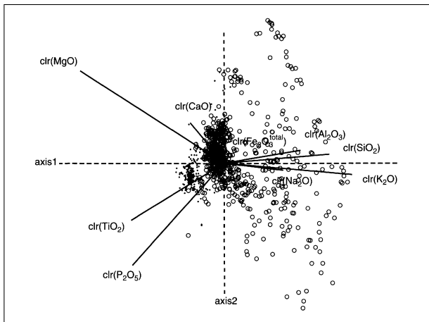
Abbildung 12: Biplot clr -transformierter Kompositionsdaten aus S^9
