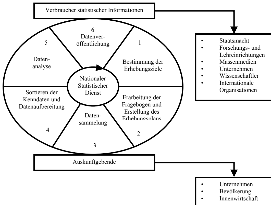
Abbildung 1: Statistisches Erhebungsschema
