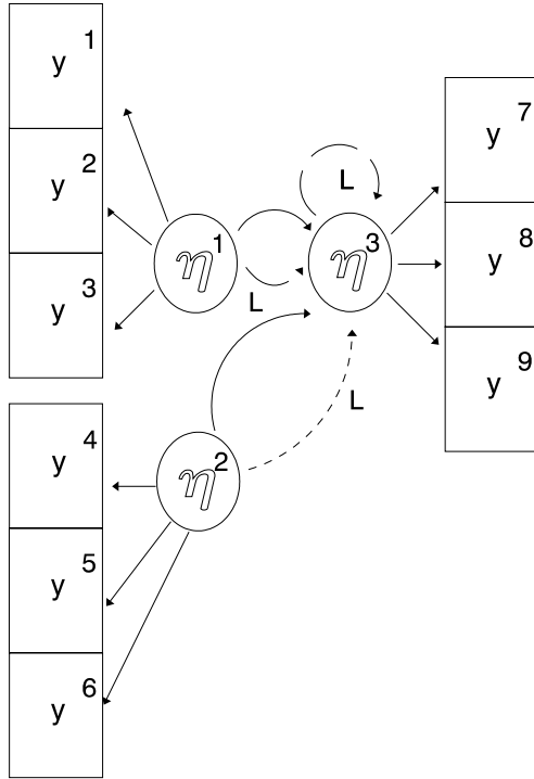
Abb. 1: Dynamisches Drei-Block-Pfadmodell
