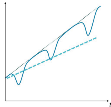
Abb. 2: Ein resilienter Pfad und ein risikoloser Pfad. Letzterer weist eine geringere durchschnittliche Wachstumsrate auf und wird langfristig vom resilienten Pfad dominiert.
