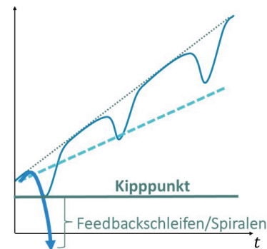
Abb. 3: Durch den Kipppunkt verliert der Pfad seine Resilienz.
