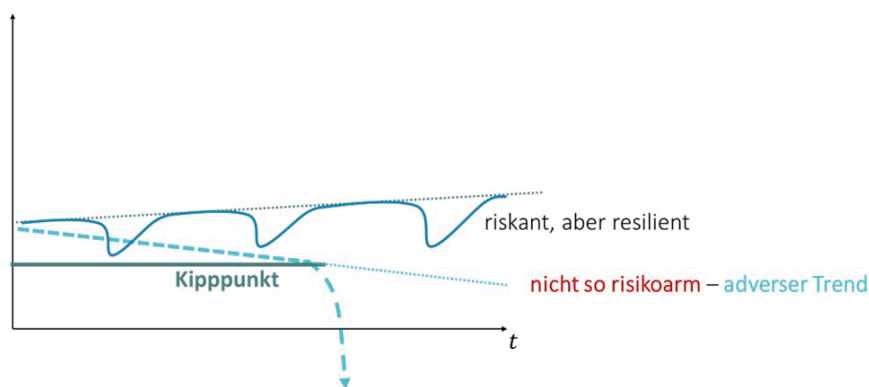
Abb. 4: Nur durch einen riskanteren, aber resilienten Pfad kann man dem Kippunkt entfliehen, da der scheinbar risikoarme Pfad einen adversen Trend aufweist.
