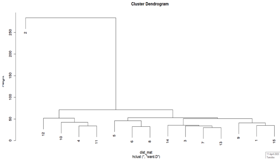
Fig. 7. Dendrogram.
