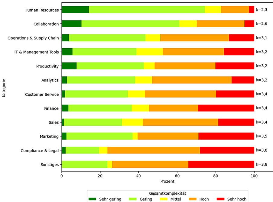
Abb. 3 Verteilung der Gesamtcomplexität und Complexitätsgrads nach Kategorien aus dem MS Power Apps AppSource
