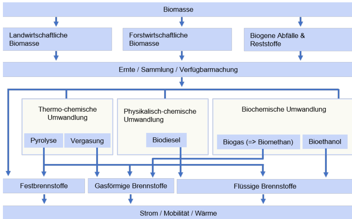
Abbildung 2: Überblick Bioenergieanlagen (eigene Darstellung, basierend auf Kaltschmitt 2024a)
