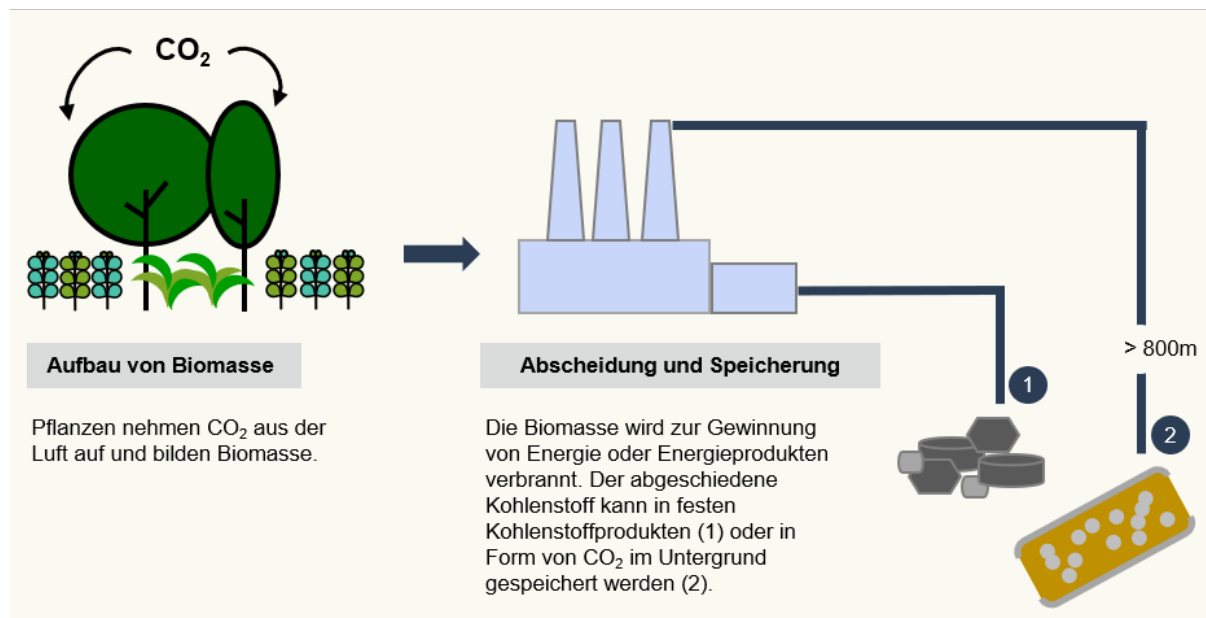
Abbildung 1: Überblick BECCS (eigene Darstellung, basierend auf Sielemann/Helmholtz SynCom, unv.)
