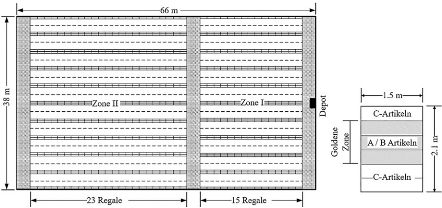
Abb. 2 Lagerlayout und Regaleinheiten
