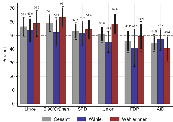
Abb. 3 Frauenanteil unter gewählten Kandidat*innen in offener Listenwahl, nach gewählter Partei und Wähler*innengeschlecht, mit 90 % und 95 %-Konfidenzintervall. N = 1320 (Linke: 102 Frauen (F), 93 Männer (M), 195 Gesamt (G); Grüne: 142 F, 84 M, 226 G; SPD: 136 F, 120 M, 256 G; Union: 118 F, 157 M, 275 G; FDP: 81 F, 49 M, 130 G; AfD: 94 F, 144 M, 238 G)
