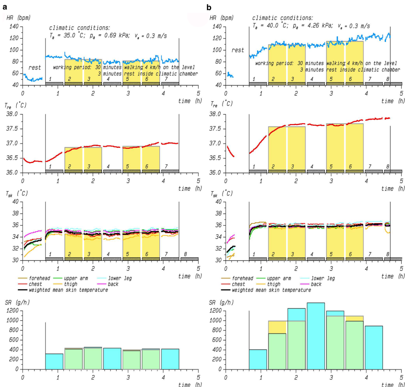
Fig. 2 Example of the development of heart rates (HR), rectal ( T_{re} ) and skin temperatures ( T_{sk} ), and sweat rates (SR) of a semi-nude, acclimated participant in heat stress exposures under warm-dry (a) and hot-humid (b) conditions, respectively. The yellowish shaded areas mark the time intervals averaged for comparing values after 1 h with those during the third hour of exposure with bar heights corresponding to the mean values Abb. 2 Zeitliche Entwicklung der Herzschlagfrequenzen (HR), Rektal- ( T_{re} ) und Hauttemperaturen ( T_{sk} ) sowie Schweißraten (SR) eines unbedeckten ( I_{cl}=0.1 clo: Shorts, Socken und Turnschuhe), akklimatisierten Probanden unter trocken-warmer (a) bzw. feucht-heißer (b) Hitzebelastung in der Klimakammer. Gelblich eingefärbte Abschnitte markieren die Zeitintervalle, die für den Vergleich der Werte nach einer Stunde mit den in der dritten Stunde registrierten Werten herangezogen werden, wobei die Höhe der Rechtecke dem Mittelwert entspricht
