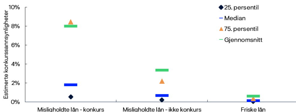
Figur 8: Estimerte konkurssannsynligheter for foretak som misligholder uten at de går konkurs, er høyere enn for foretak med friske lån
