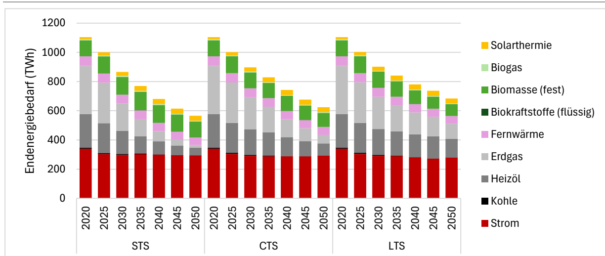
Abbildung 2: Entwicklung des Endenergiebedarfs des deutschen Gebäudesektors
