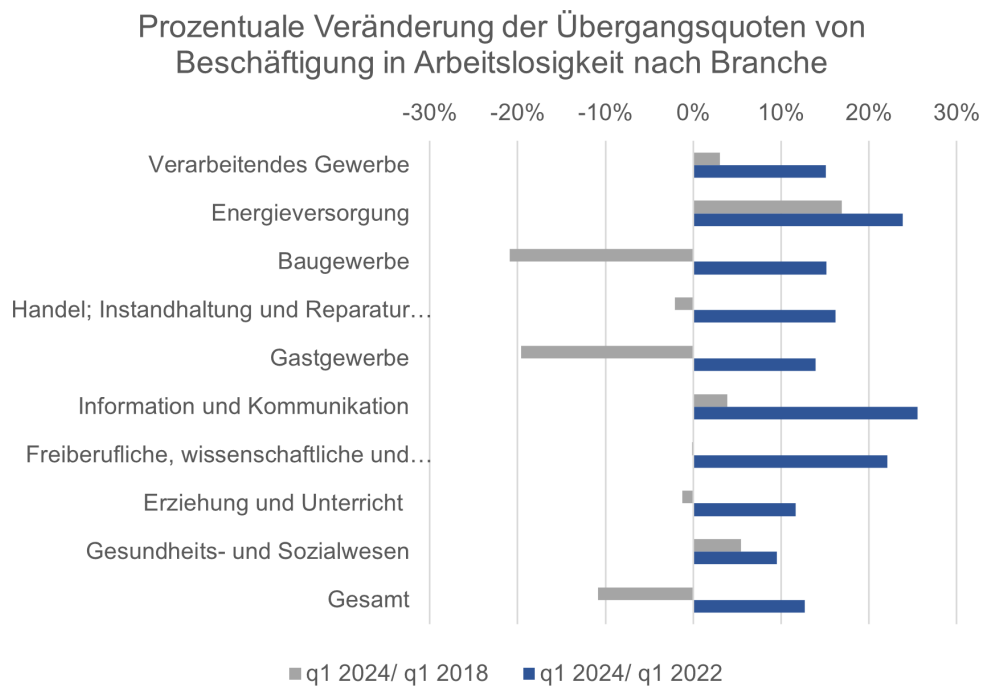
Abbildung 4 Veränderung Zugangsrisiko
