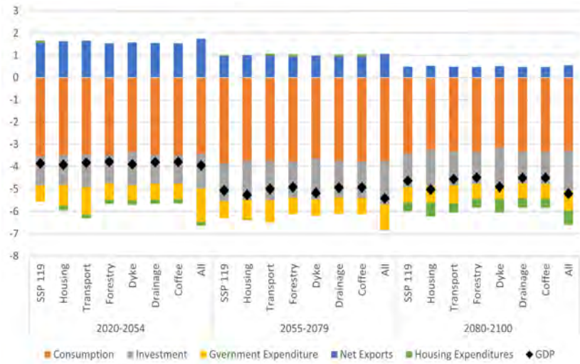
SSP 245
