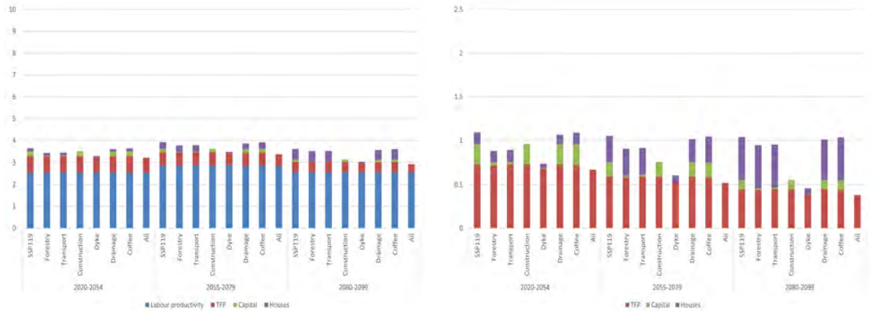
SSP 245
