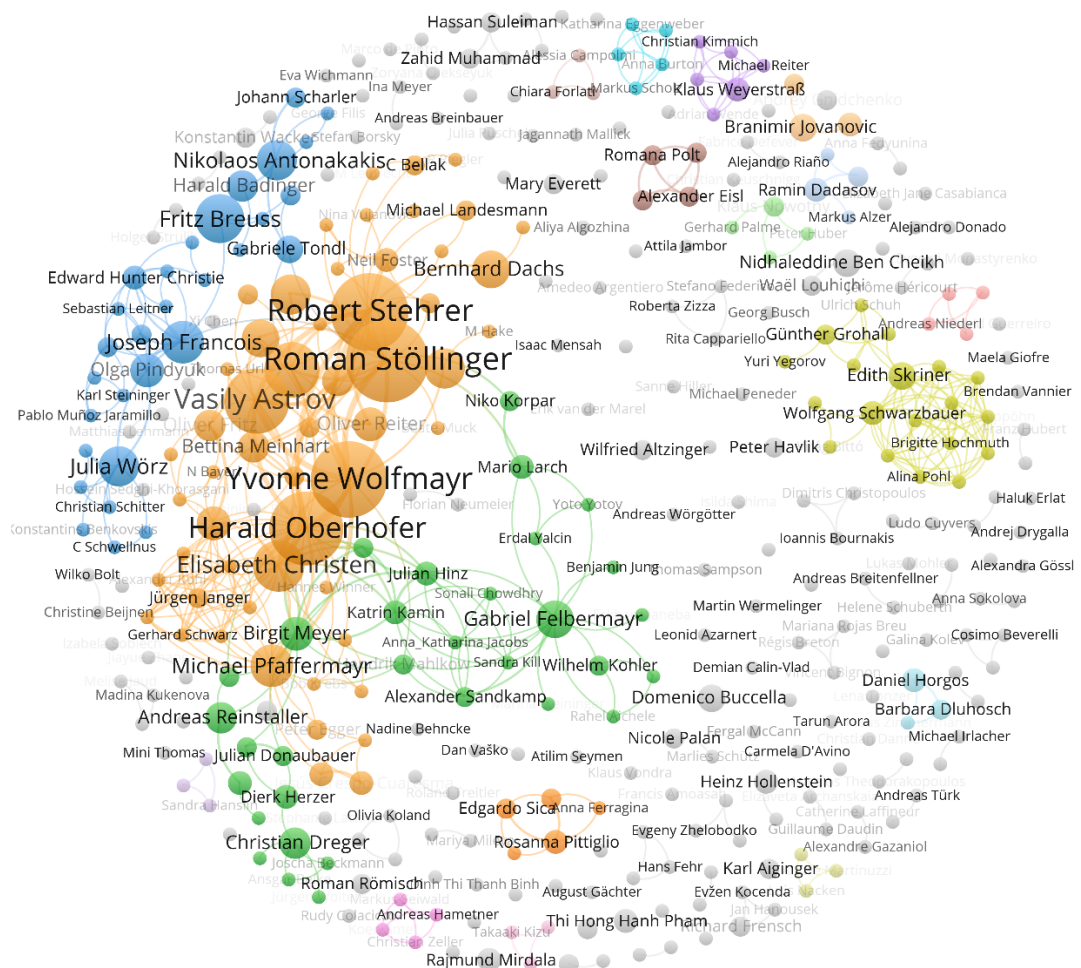
Abbildung 26: Uneingeschränktes Autorennetzwerk
