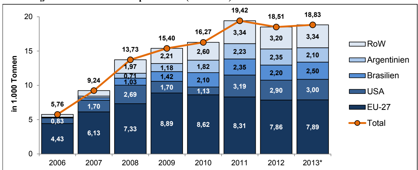
Abbildung 8. Weltweite Biodieselproduktion (2006-2013)
