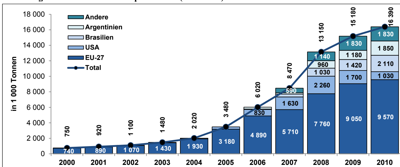
Abbildung 8. Weltweite Biodieselproduktion (2000-2010)
