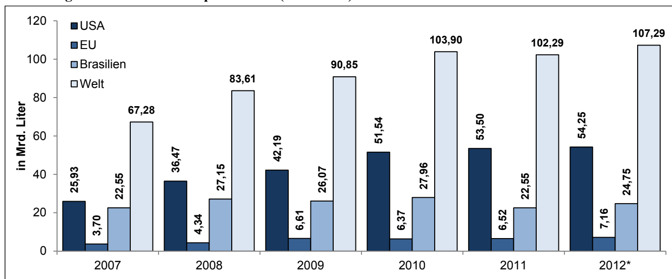
Abbildung 10. Globale Ethanolproduktion (2007-2012)
