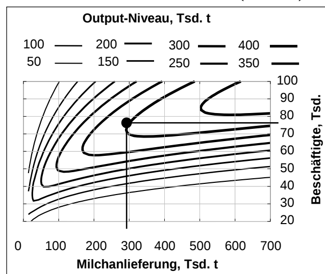
Abbildung 2. Ermittelte Isoquanten der Translog-Produktionsfunktion (Modell I)
