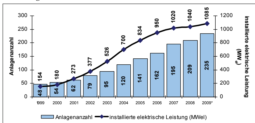
Abbildung 10. Biomasseheizkraftwerke
