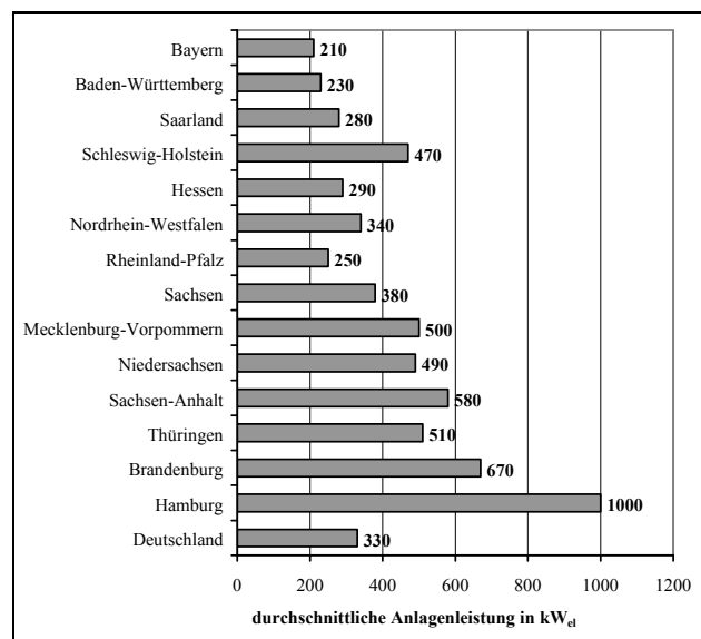
Abbildung 7. Durchschnittliche Anlagenleistung im Jahr 2008
