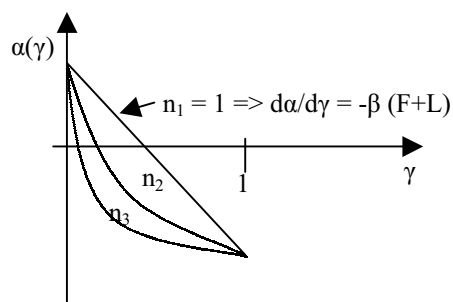
Anteil der schadhafte Einheiten \alpha(\gamma) in Abhängigkeit von der Kontrollintensität \gamma bei unterschiedlicher Anzahl n der erzeugten Partien je Hersteller
