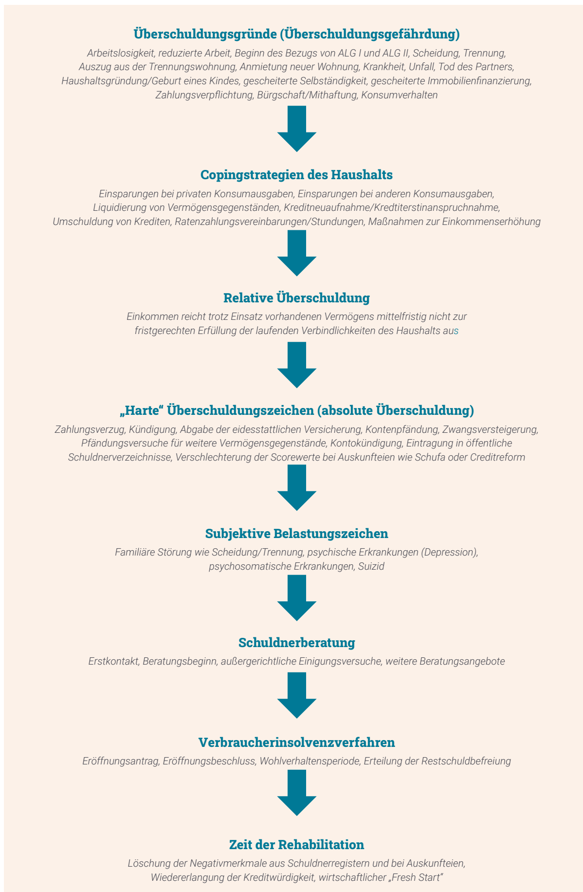
Abbildung 1: Typischer Überschuldungsverlauf
