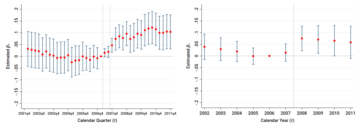
(a) LEHD
