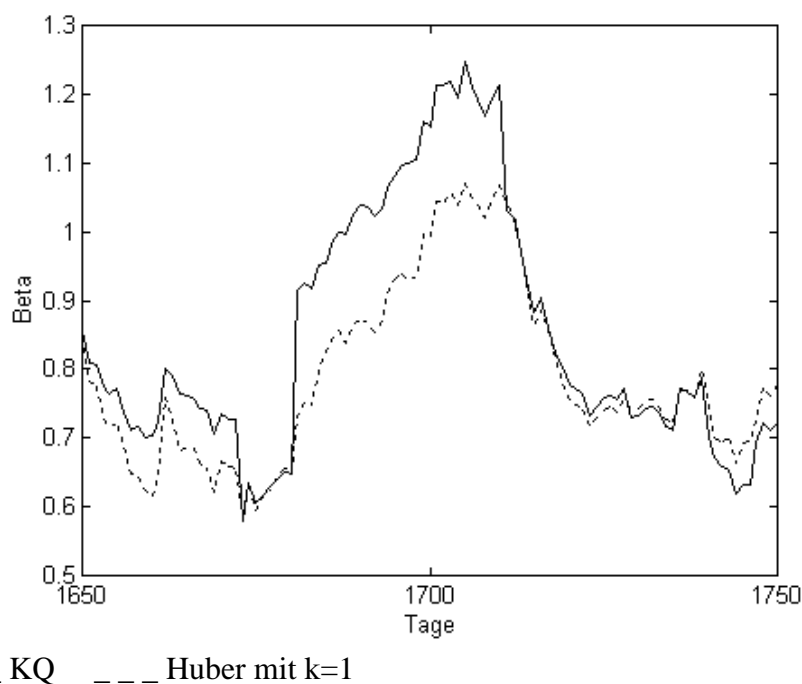
Abb. 4: Die 30-Tages-Betafaktoren von VEBA von Tag 1650 bis 1750
