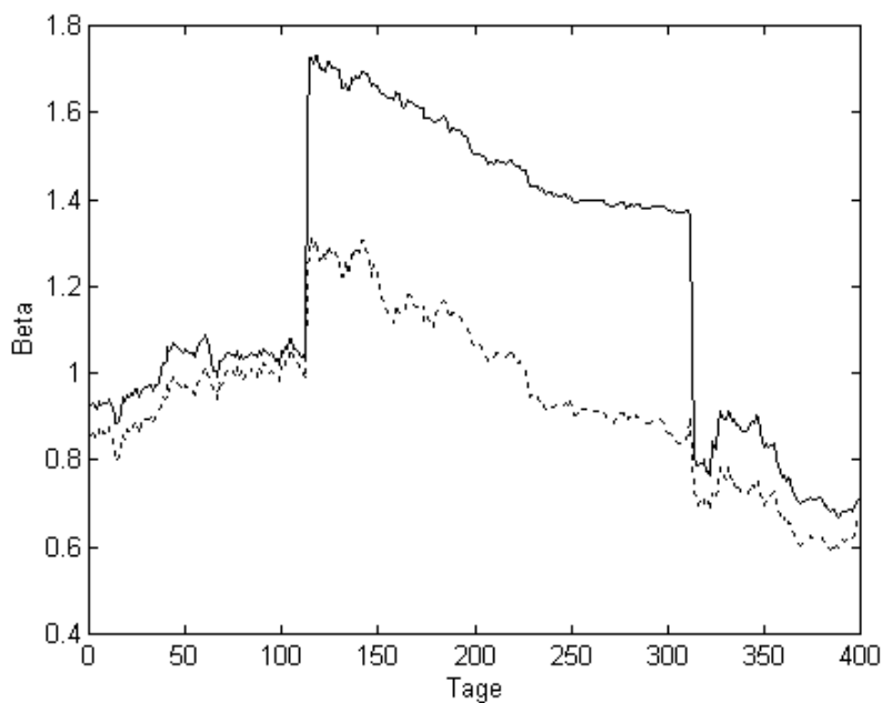
Abb. 7: Die 30-Tages-Betafaktoren der Metallgesellschaft von Tag 1 bis 400
