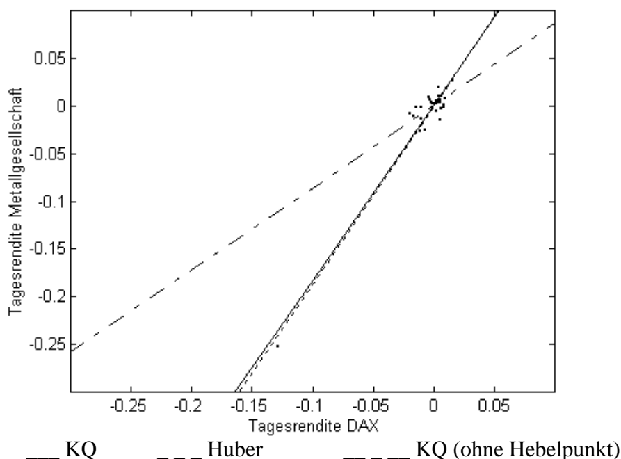
Abb.9: Die Entstehung der KQ- und M-Regressionsgerade der Metallgesellschaft am Tag 113
