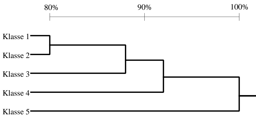
Abb. 7: Dendrogramm
